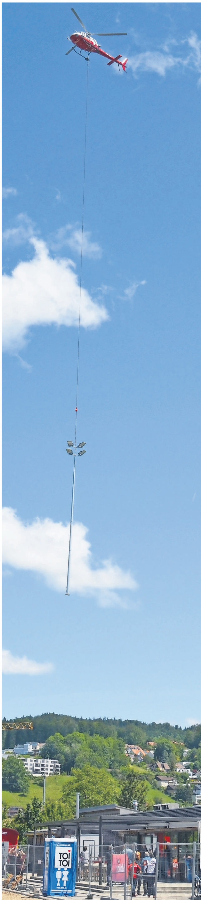
Der Lichtmast wird in den vorbereiteten Sockel eingepasst.
